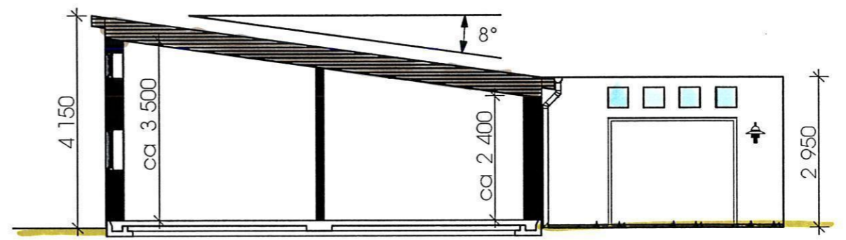
SEKTION A-A
